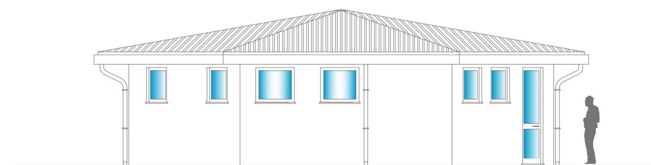
PROSPETTO LATERALE
