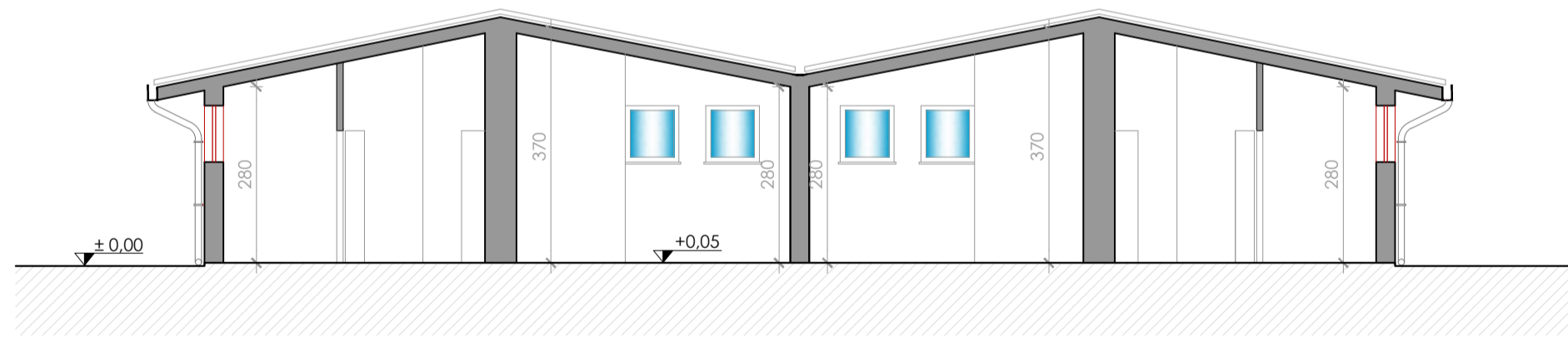
SEZIONE A-A
