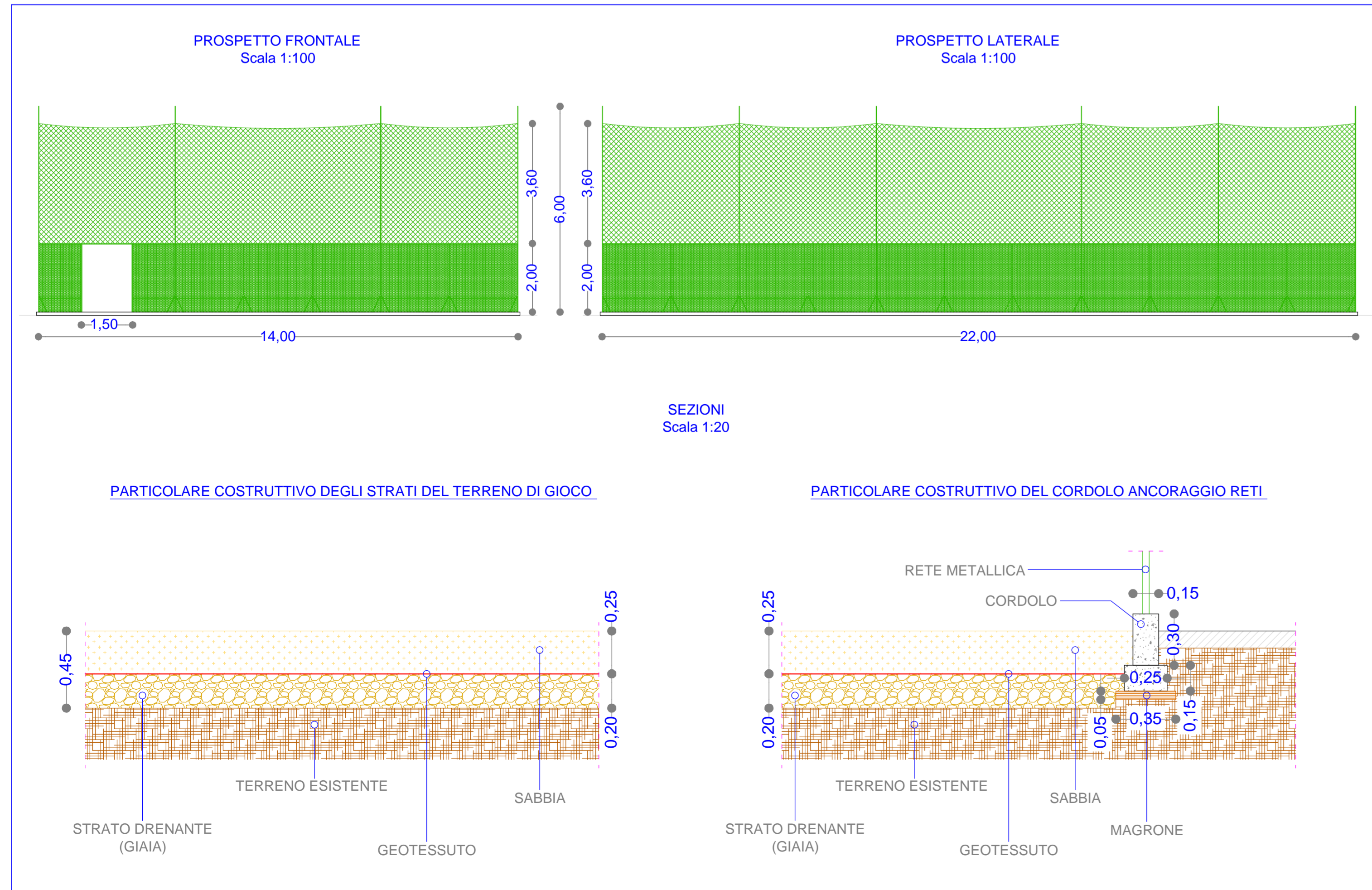
PROSPETTI E SEZIONI QUOTATE
