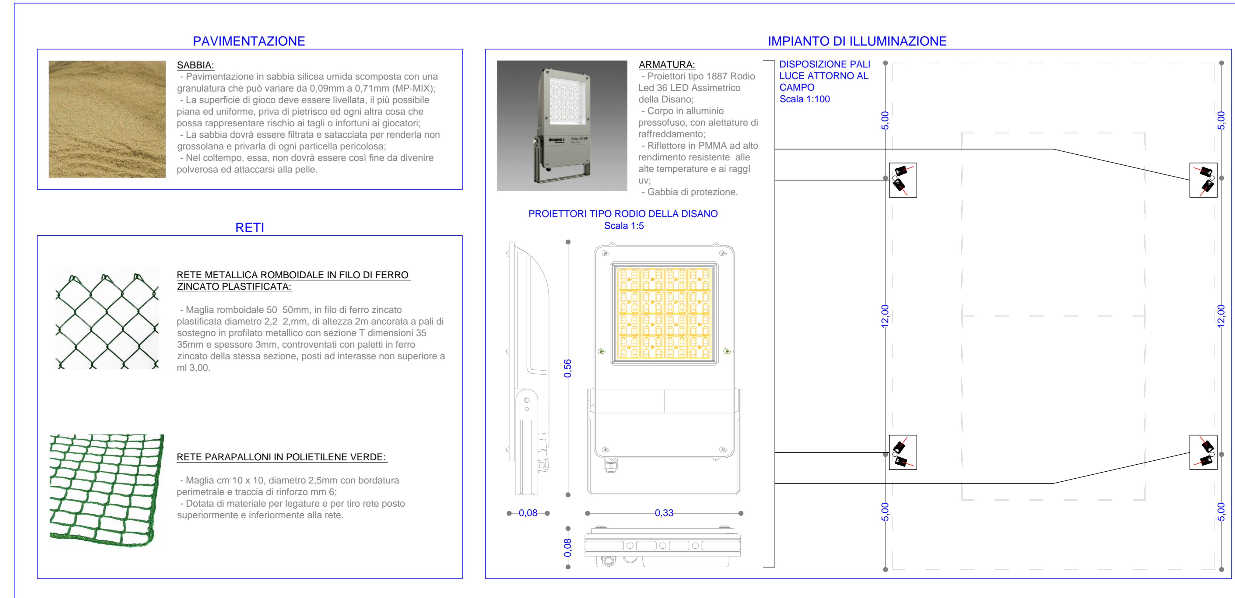
CARATTERISTICHE E TIPOLOGIE MATERIALI PER LA REALIZZAZIONE DEL CAMPO DA BEACH VOLLEY
