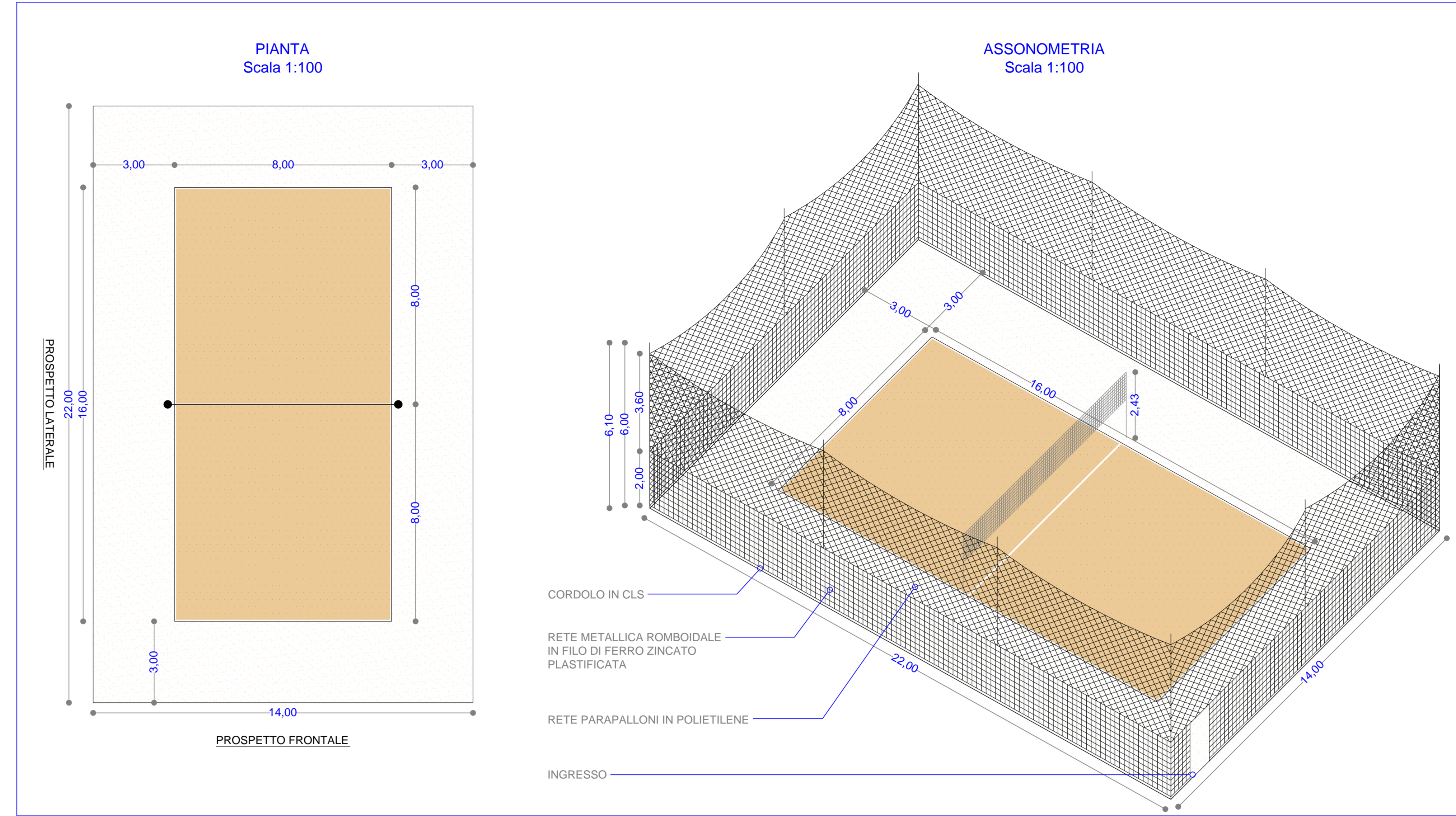
PIANTE GIOCO E ASSONOMETRIE QUOTATE
