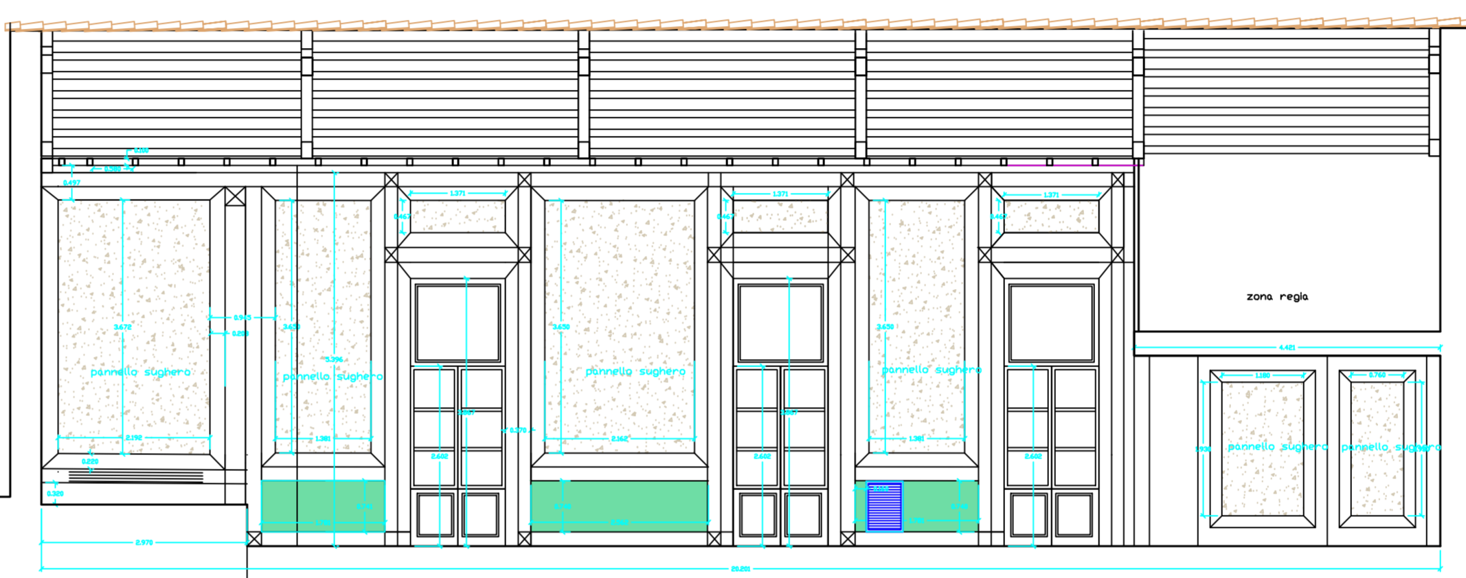
Parete D
