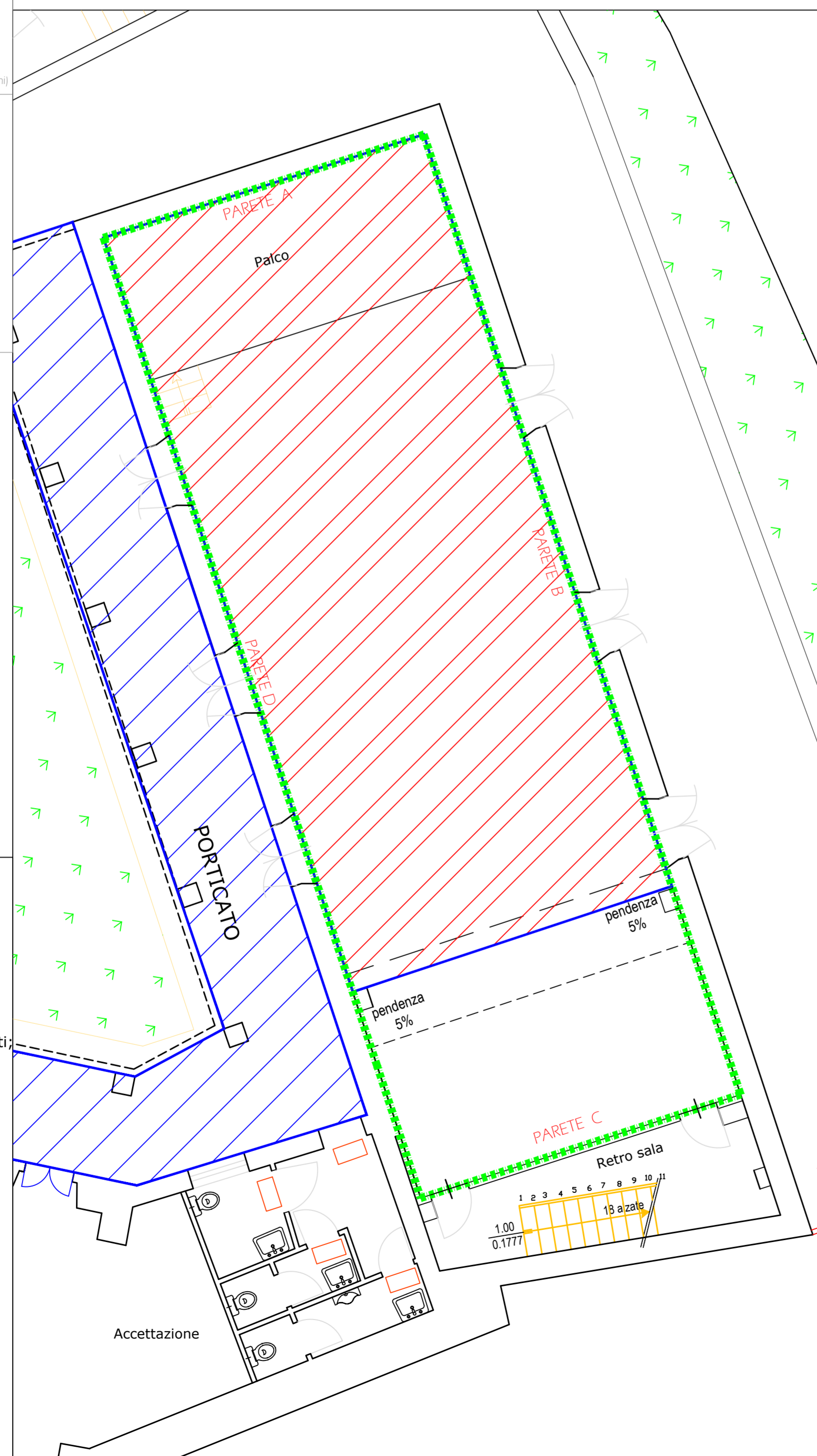
Sala Convegni Scale 1:75
