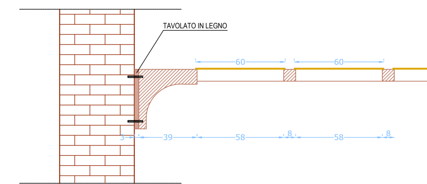
PARTICOLARE A SCALA 1:20
