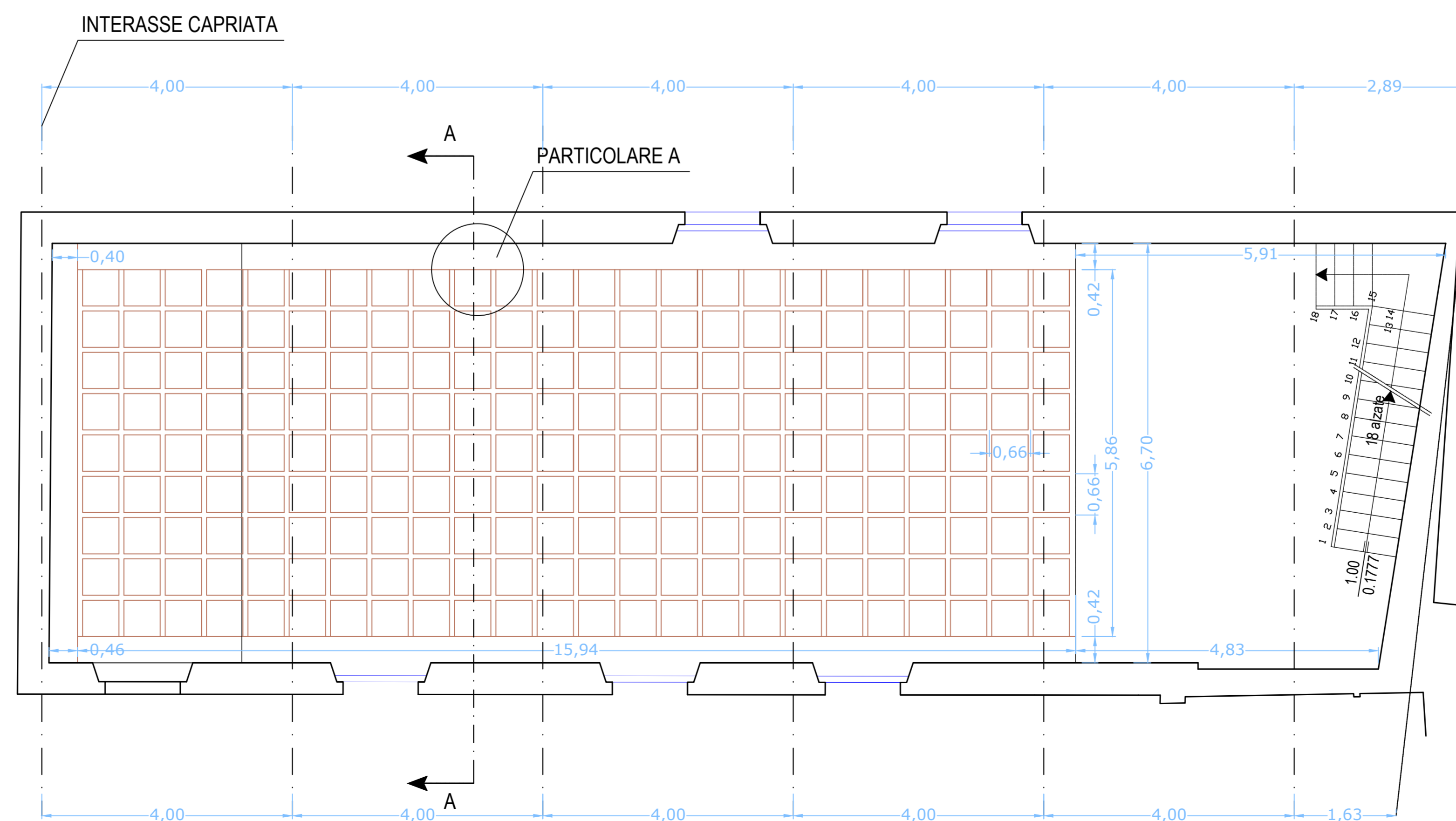
Particolare Controsoffitto Scale 1:75
