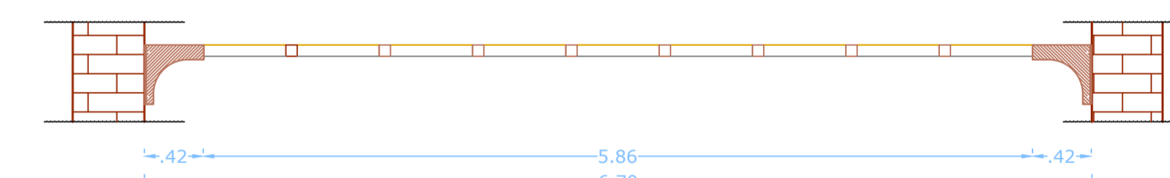
SEZIONE COPERTURA SCALA 1:50
