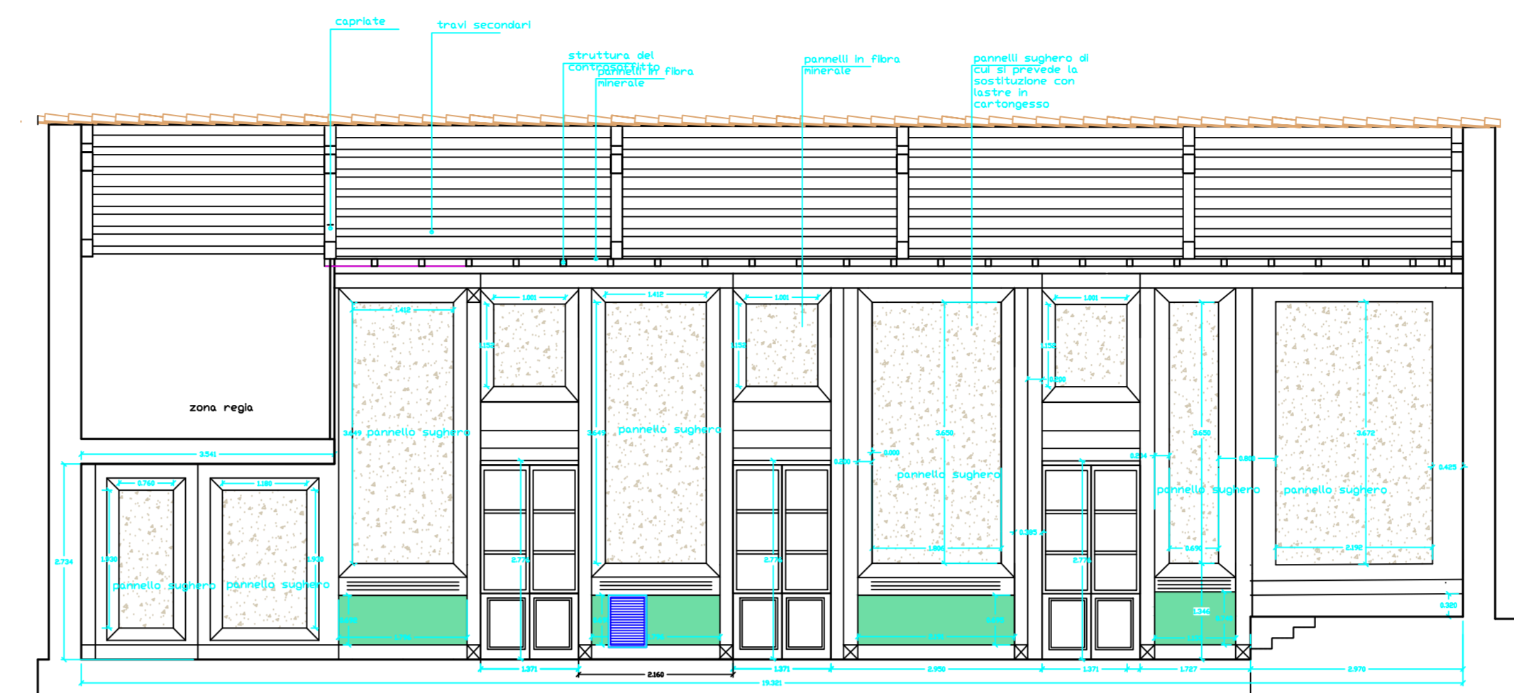
Parete B
