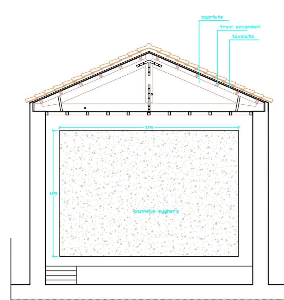
Parete A
