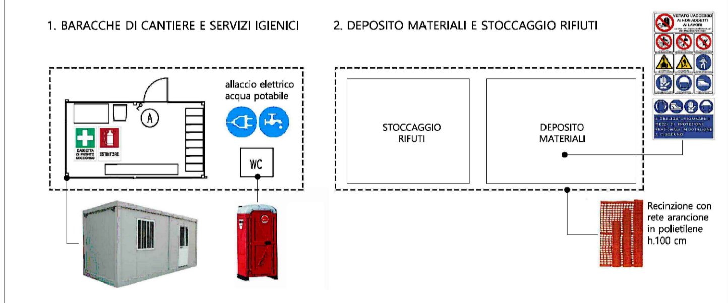
ALLESTIMENTO CANTIERE
