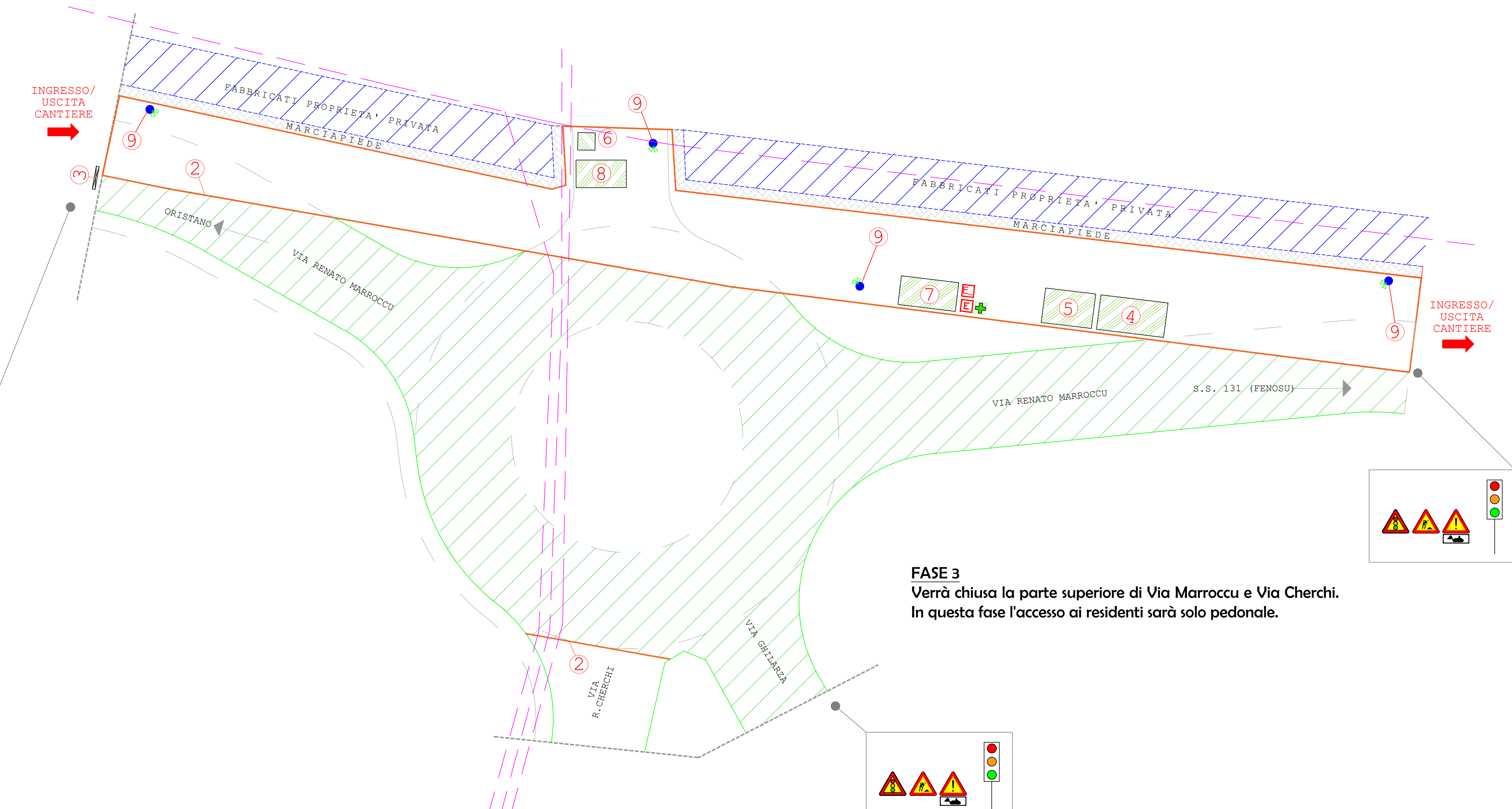
PLANIMETRIA LAYOUT DI CANTIERE FASE 3
