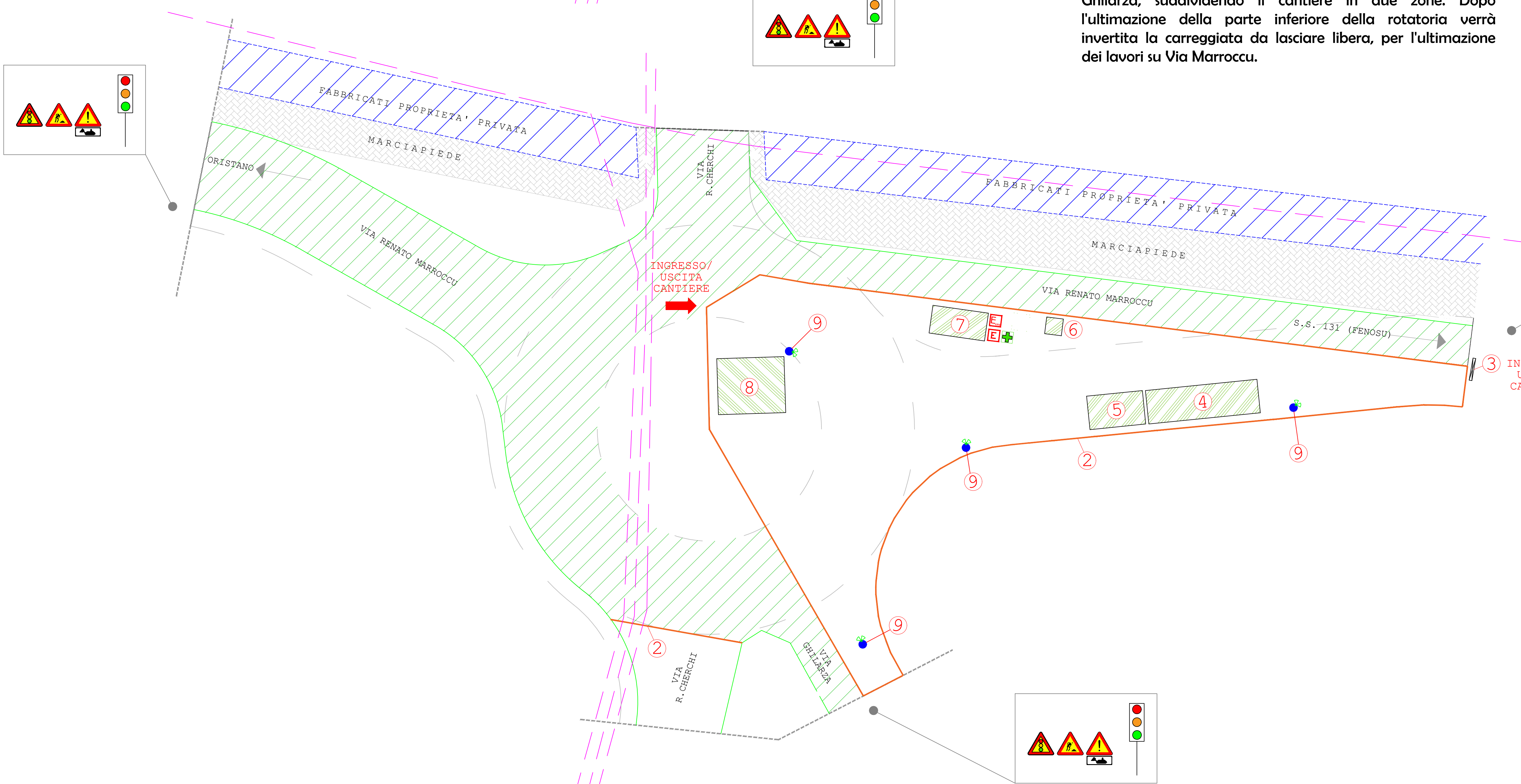
PLANIMETRIA LAYOUT DI CANTIERE FASE 2
