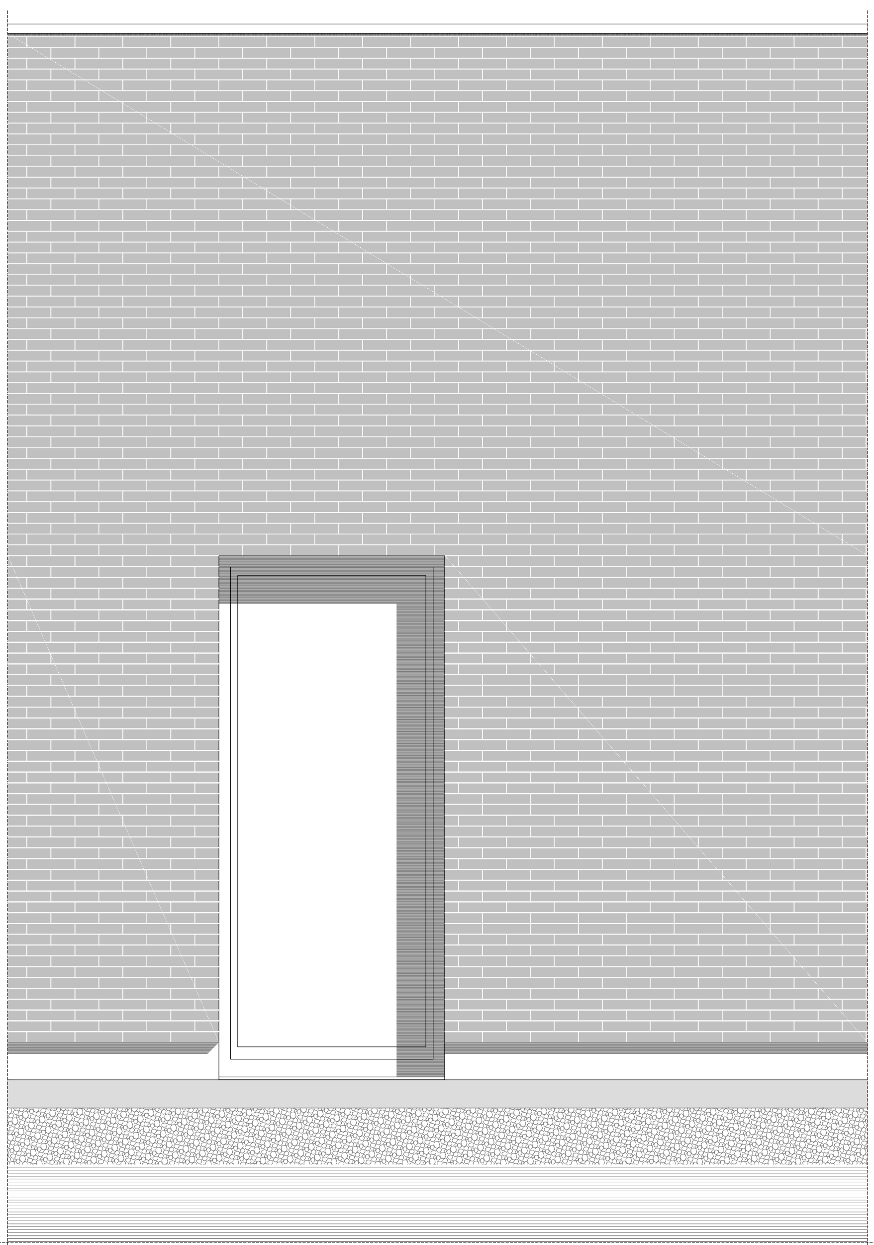
PROSPETTO ARCHIVIO scala 1:20
