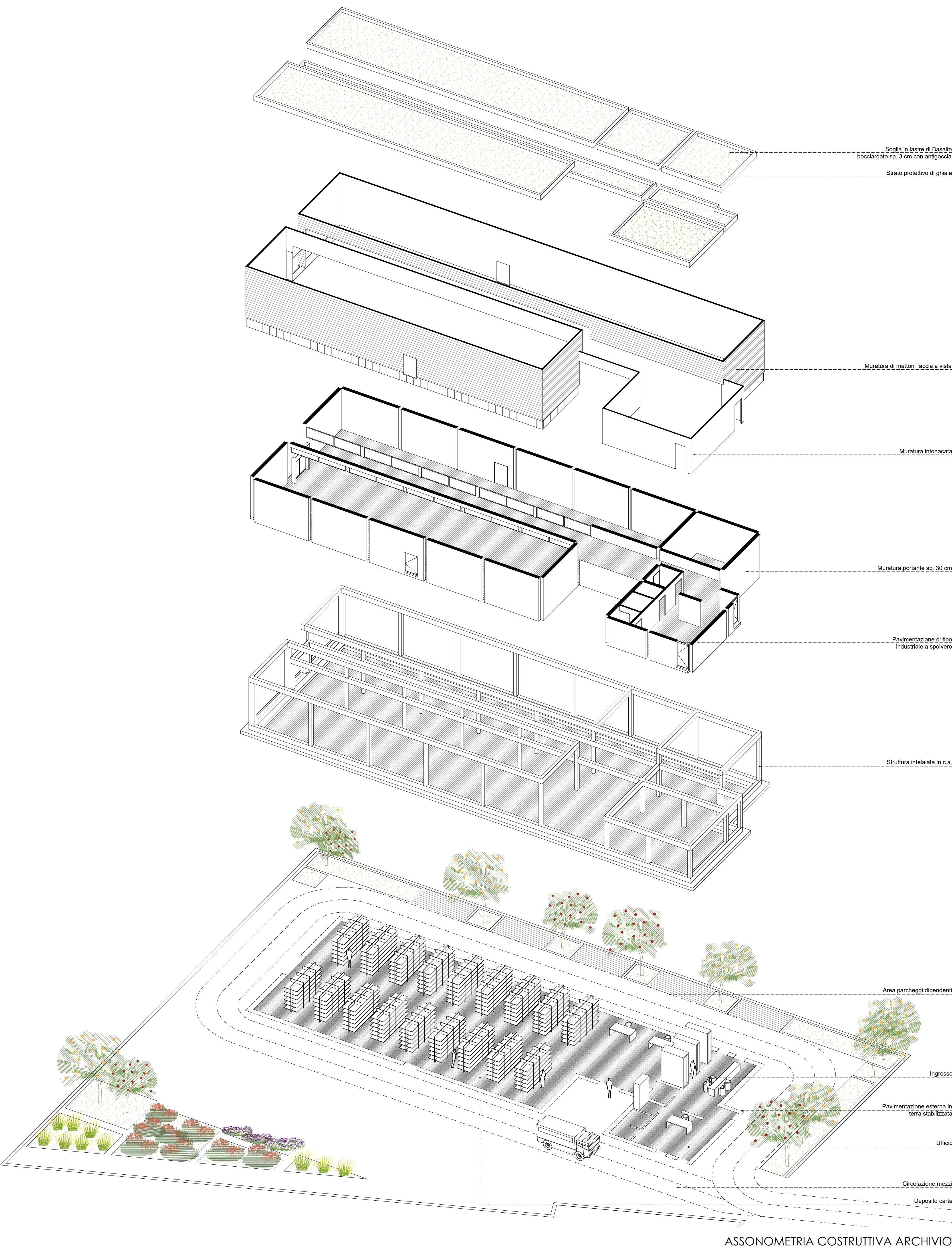
ASSONOMETRIA COSTRUTTIVA ARCHIVIO
