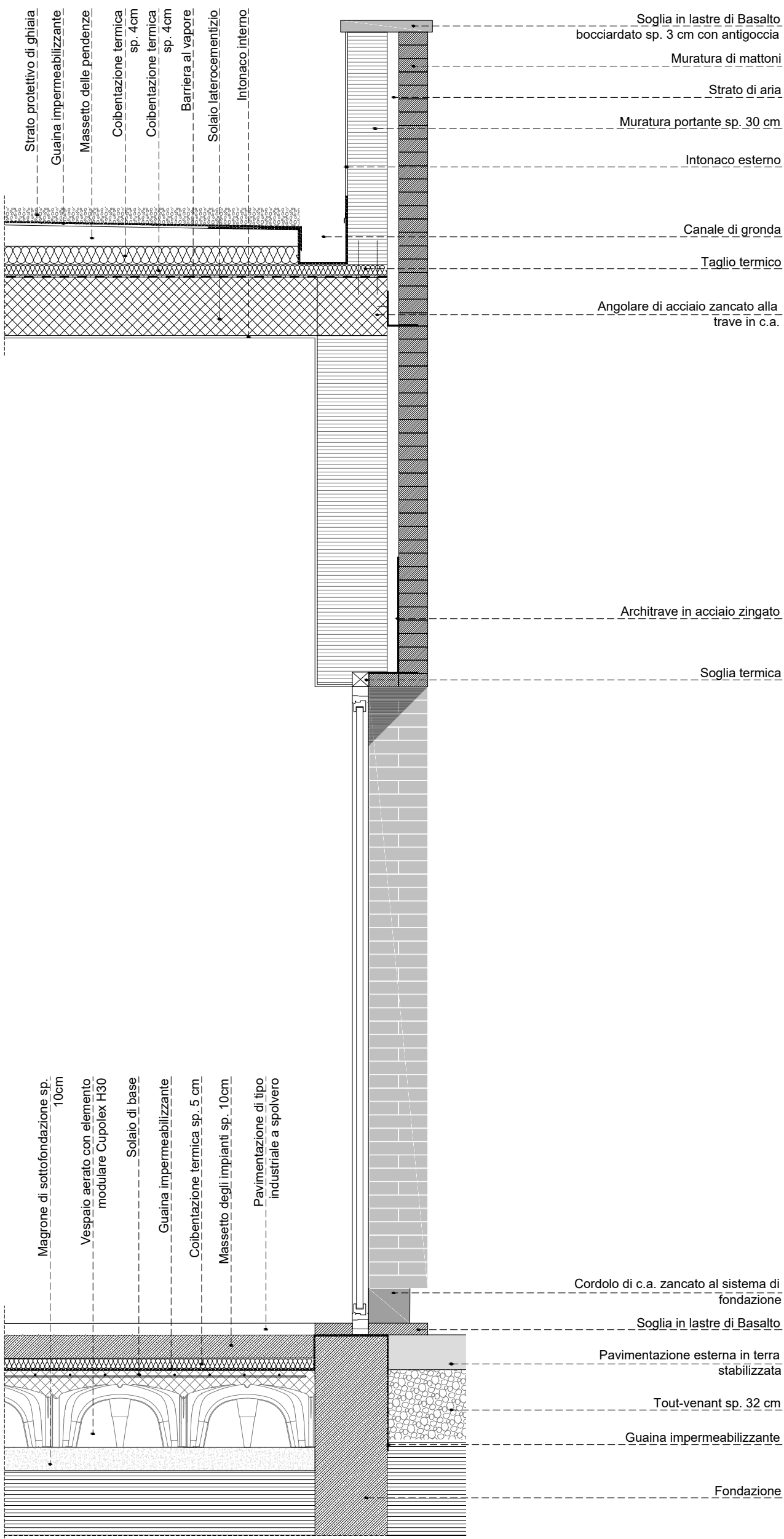
SEZIONE ARCHIVIO scala 1:20
