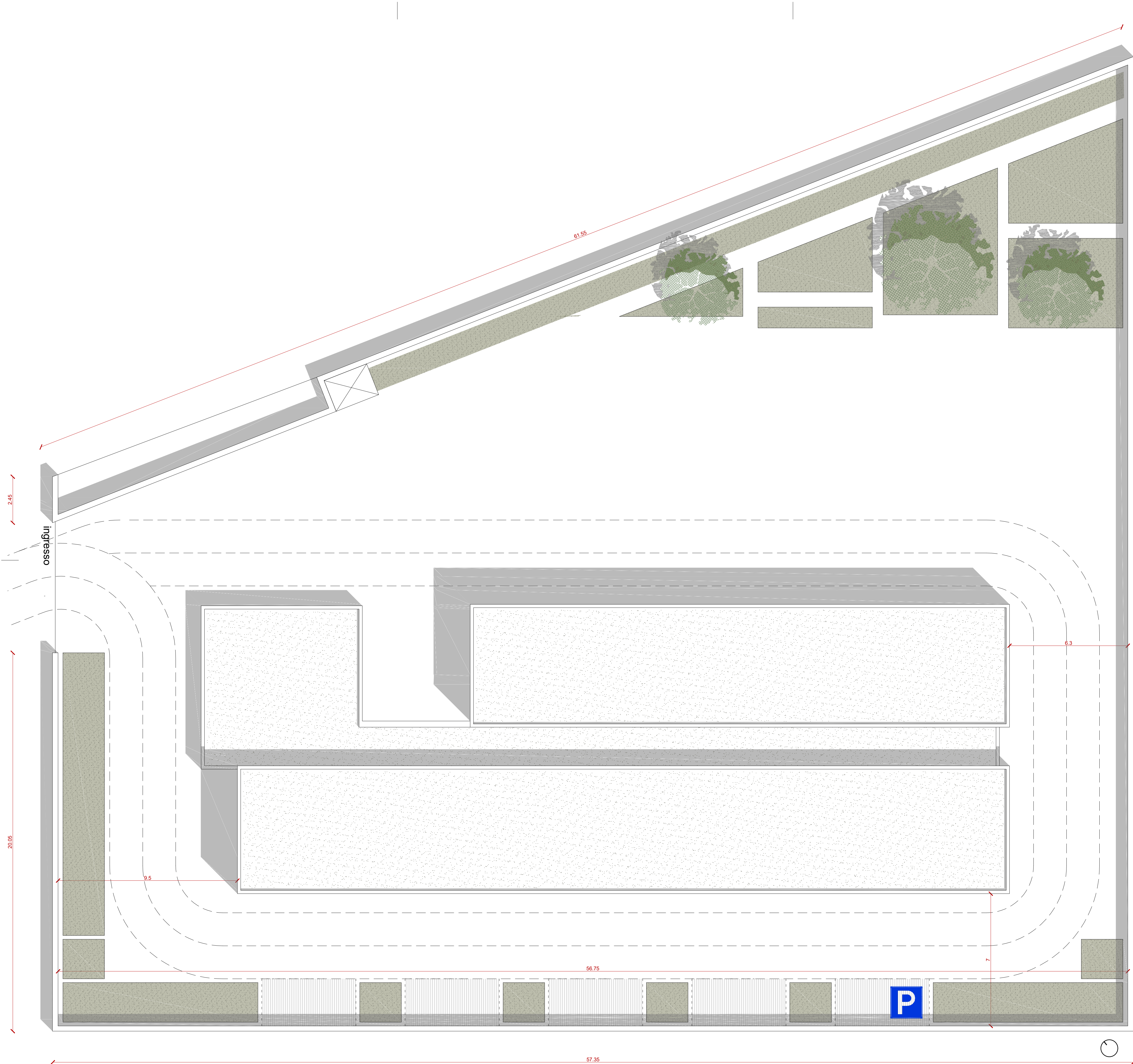
PLANIMETRIA GENERALE_SCALA 1:200
