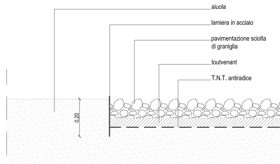
particolare divisione area verde e sentiero sc 1:10
