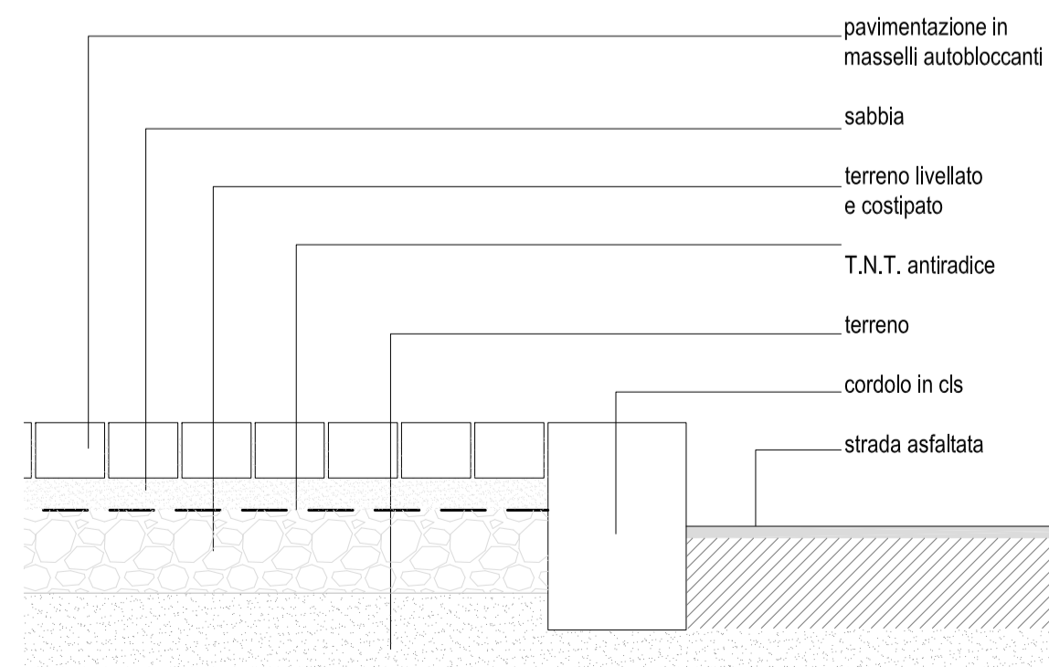
particolare pavimentazione drenante del marciapiede sc 1:10
