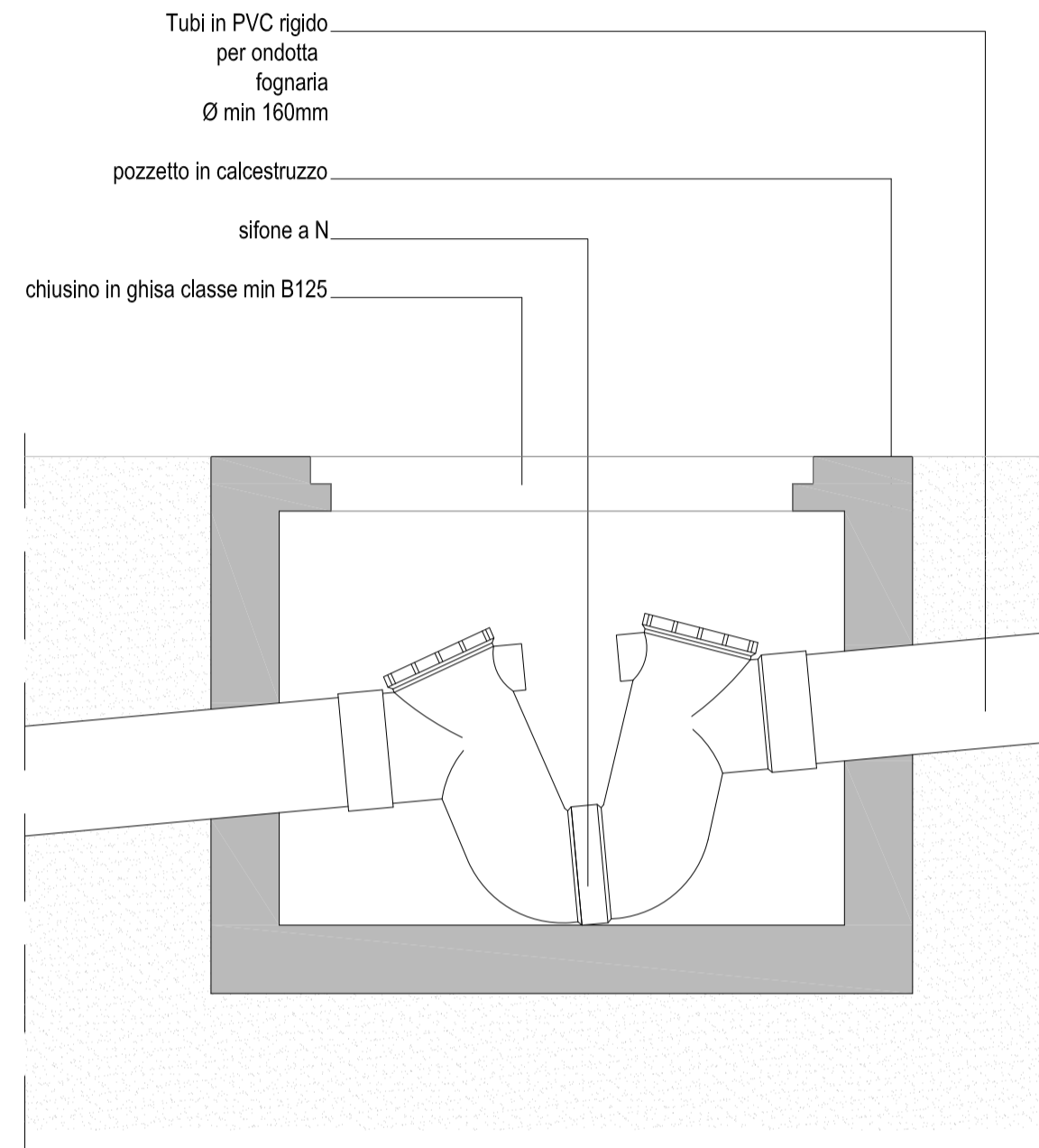
particolare pozzetto di ispezione per allaccio fognario sc 1:10
