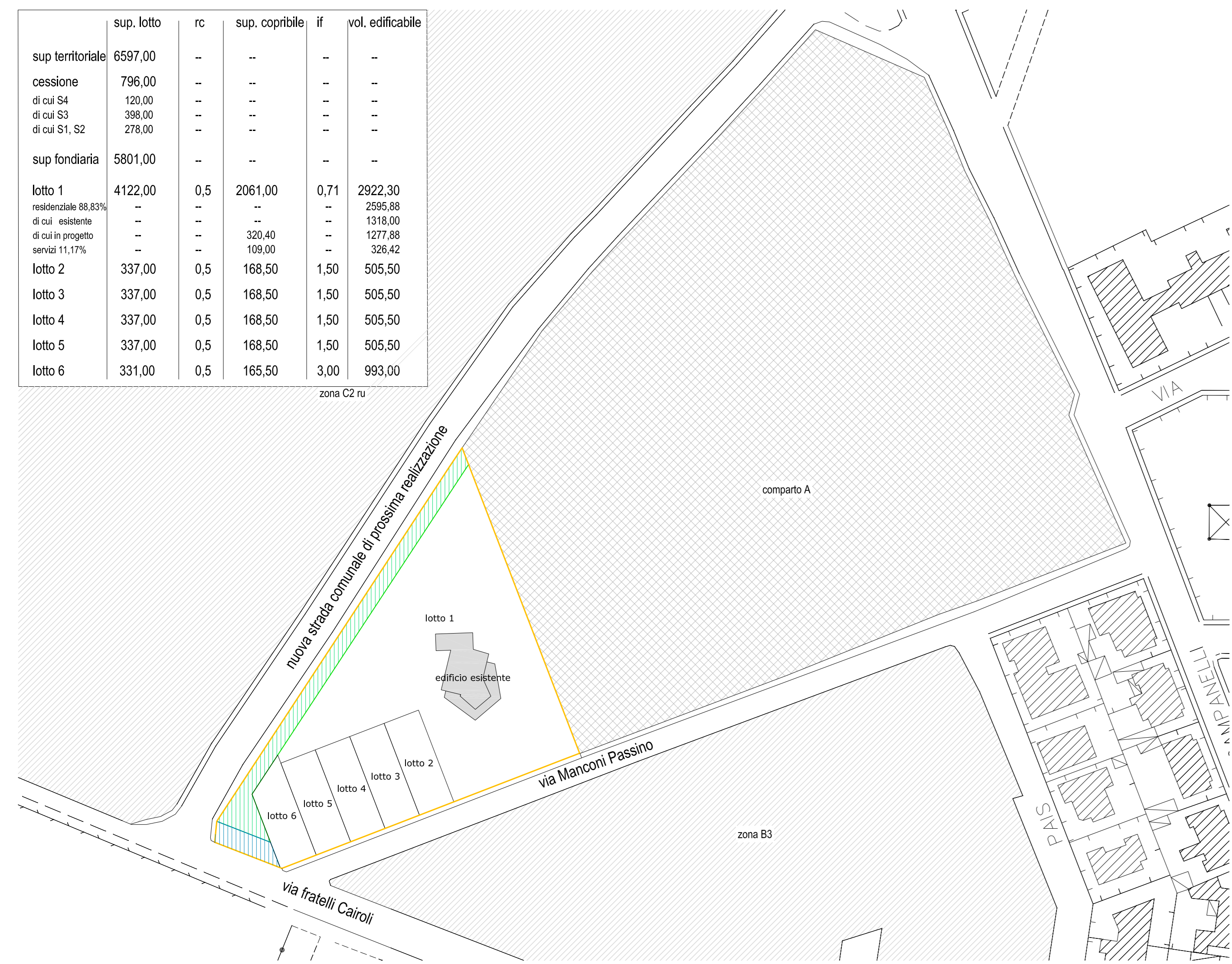
planimetria generale sc 1:1000
